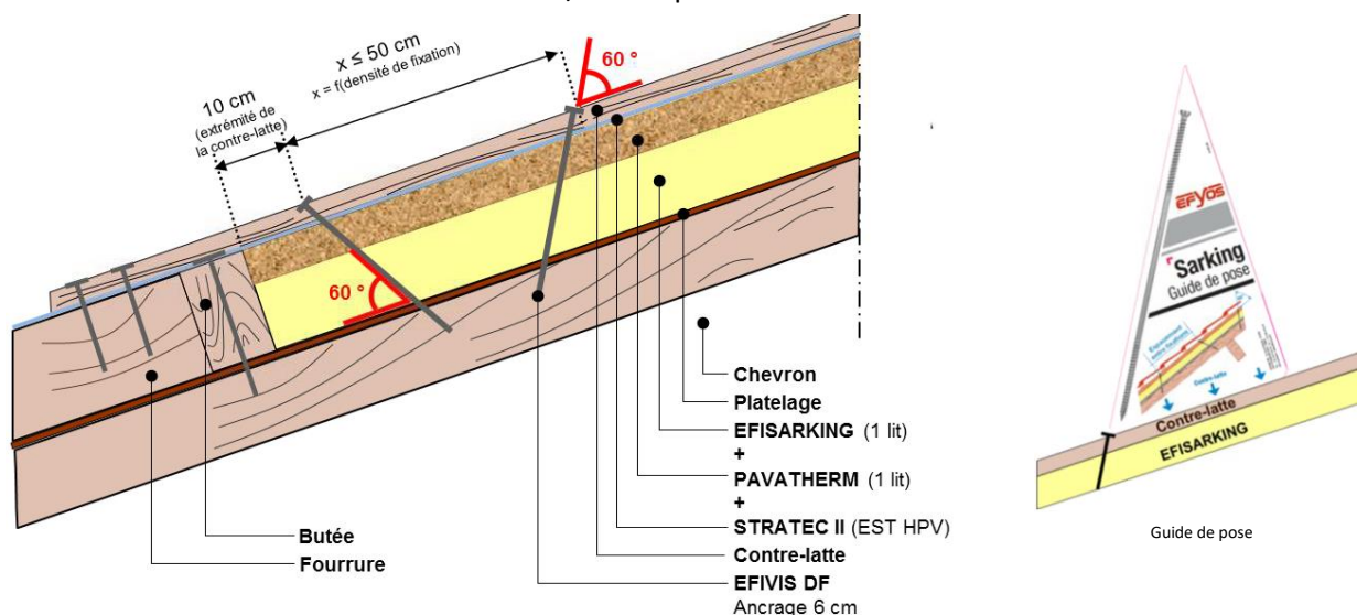
Figure 10 : Fixation des EFIVIS DF -EFISARKING épaisseur \geq 160 \text{ mm} ou EFISARKING + PAVATHERM/EST
