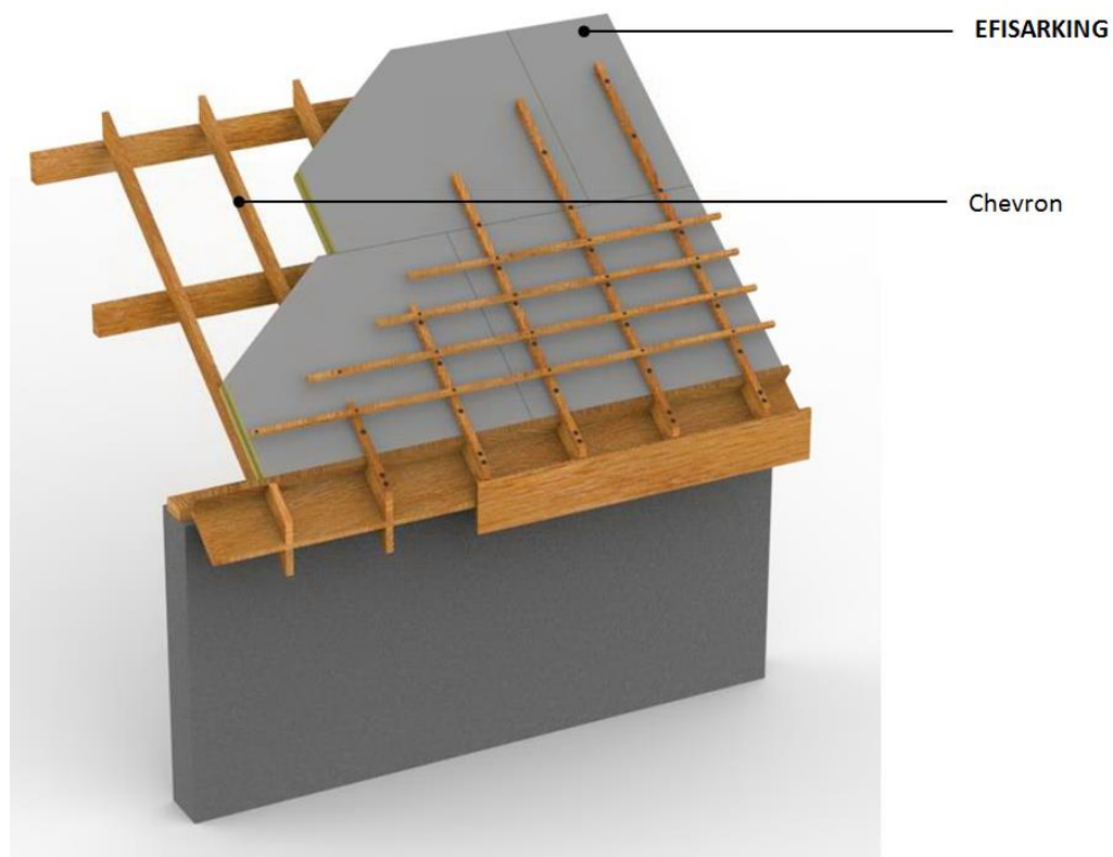
Figure 2 : Schéma de principe du procédé EFISARKING sans platelage
