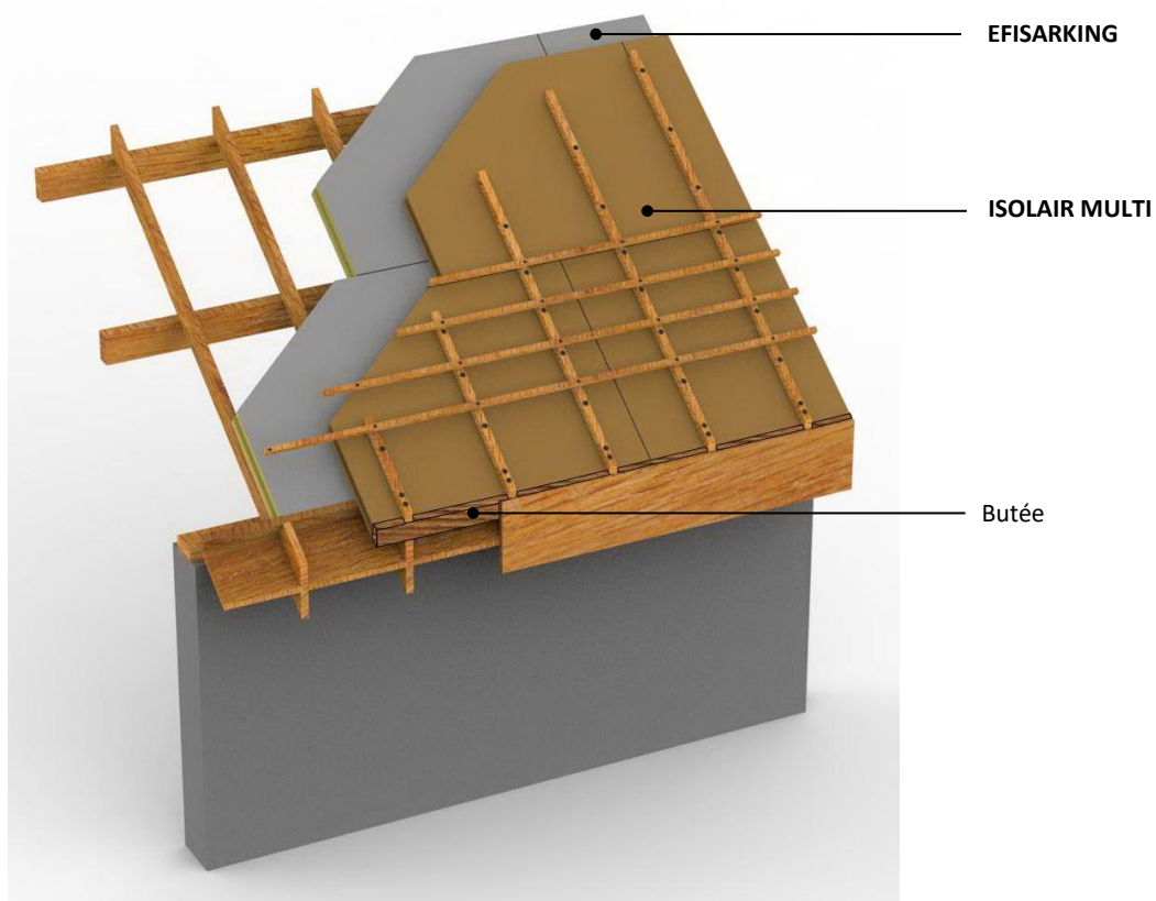
Figure 4 : Schéma de principe du procédé EFISARKING sans platelage avec panneau ISOLAIR MULTI complémentaire
