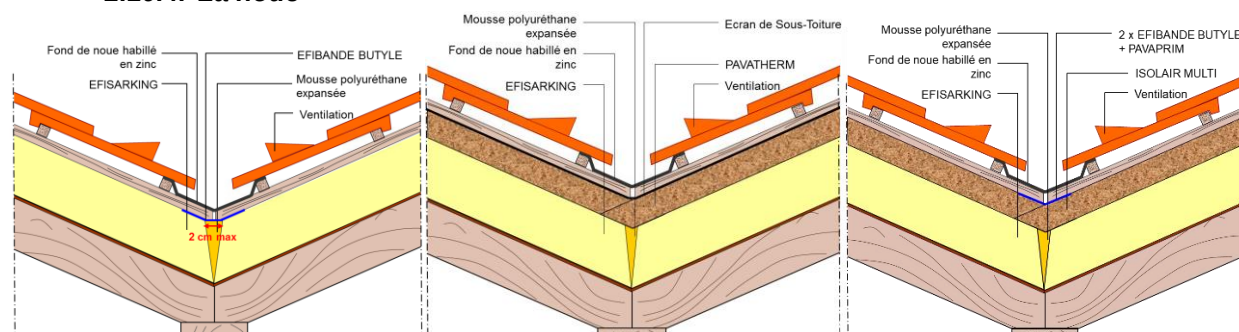
Figure 15 : Finition en noue - (de gauche à droite) EFISARKING , EFISARKING + PAVATHERM/EST , EFISARKING + ISOLAIR MULTI
