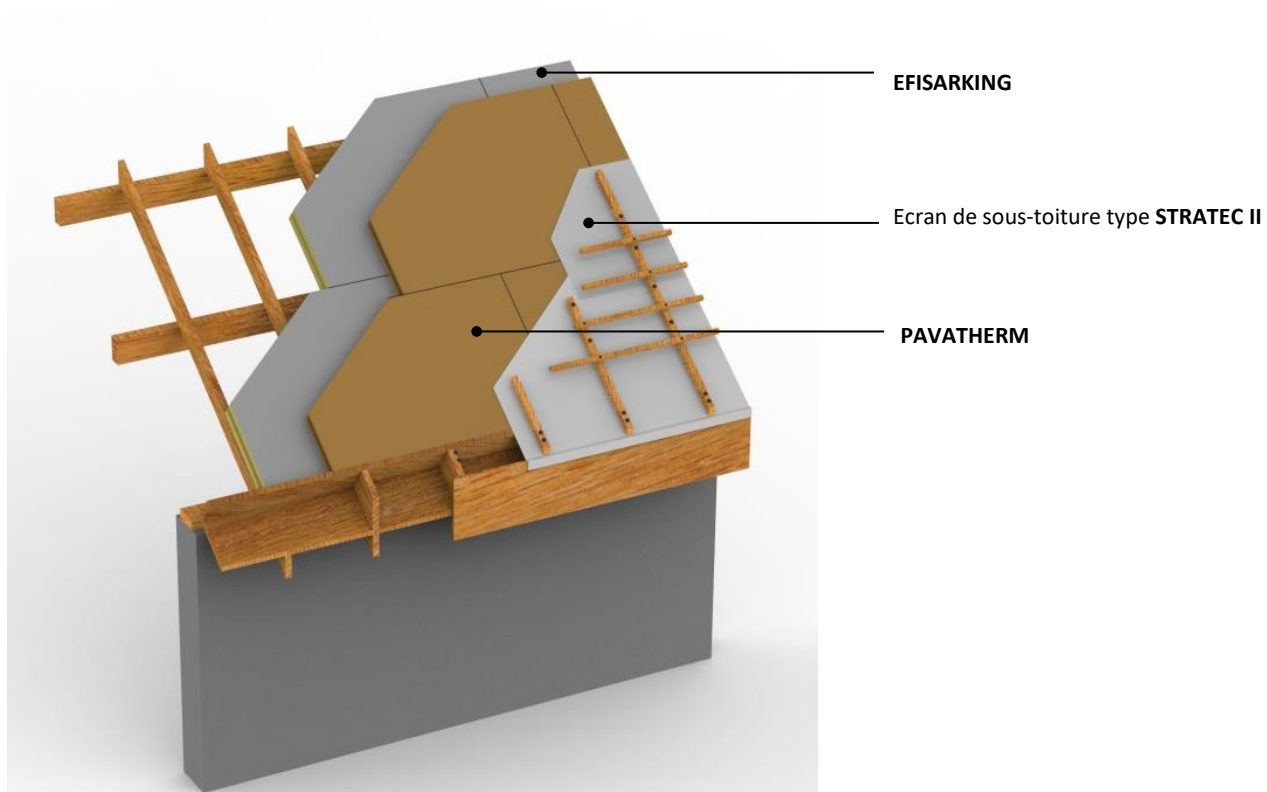
Figure 3 : Schéma de principe du procédé EFISARKING sans platelage avec panneau PAVATHERM complémentaire
