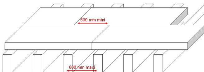
Figure 6 : Schéma de principe de la pose sans platelage de l'isolant thermique
