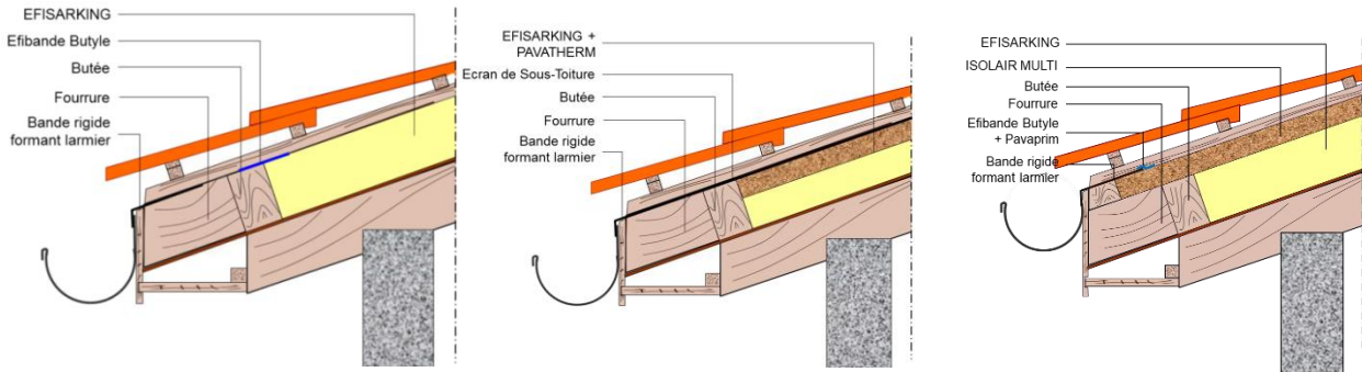
Figure 12 : Finition à l'égout - (de gauche à droite) EFISARKING , EFISARKING + PAVATHERM/EST , EFISARKING + ISOLAIR MULTI
