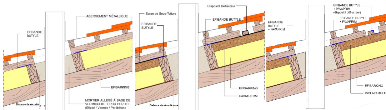
Figure 19 : Traitement d'un abergement - (de gauche à droite) EFISARKING , EFISARKING + PAVATHERM/EST , EFISARKING + ISOLAIR MULTI
