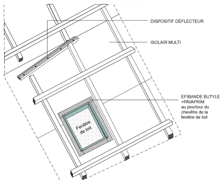
Figure 17: Dispositif deflecteur sur panneau ISOLAIR MULTI
