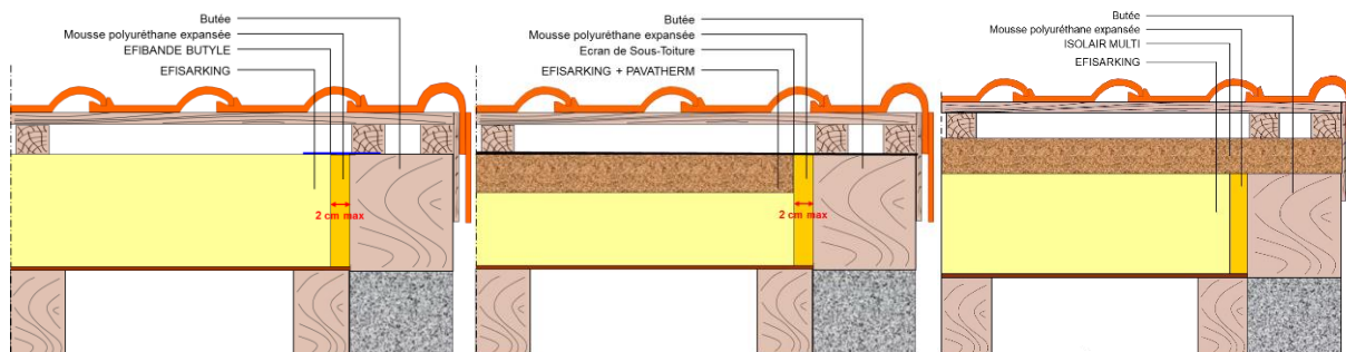
Figure 14 : Finition en rive latérale - (de gauche à droite) EFISARKING , EFISARKING + PAVATHERM/EST , EFISARKING + ISOLAIR MULTI
