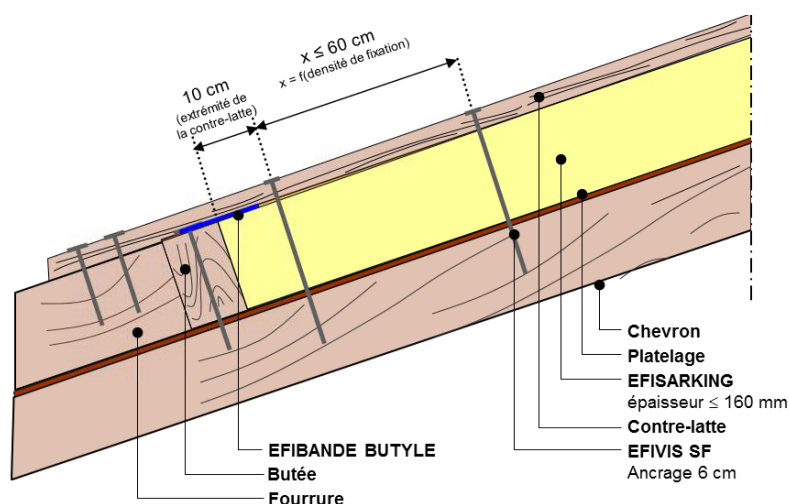
Figure 9 : Fixation des EFIVIS SF - EFISARKING épaisseur \leq 160 mm
