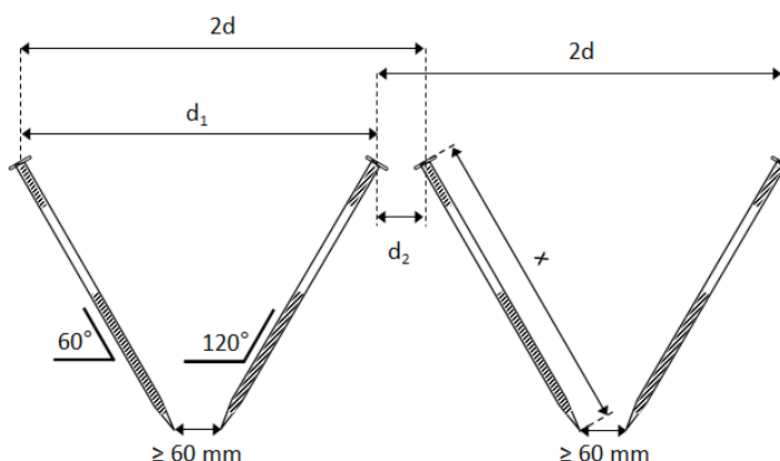
Figure 20 - Distance entre fixations EFIVIS DF
