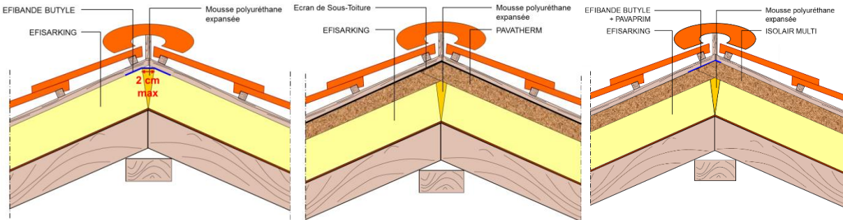
Figure 13 : Finition au faîtage - (de gauche à droite) EFISARKING , EFISARKING + PAVATHERM/EST , EFISARKING + ISOLAIR MULTI
