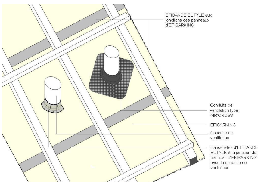
Figure 18 : Traitement d'une sortie de ventilation
