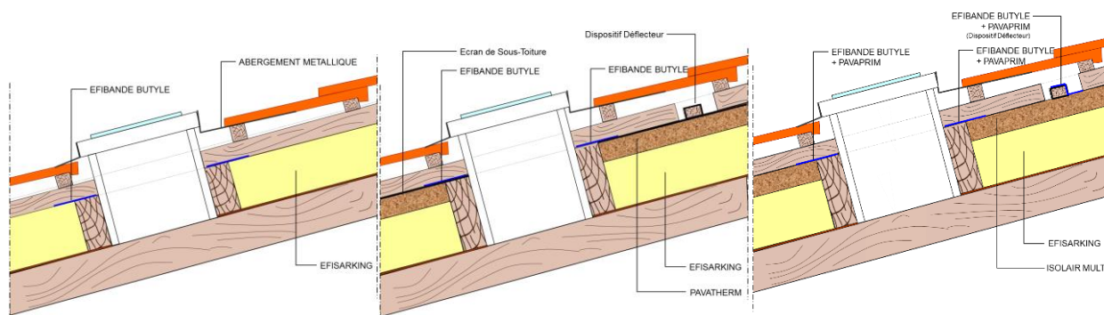
Figure 16 : Traitement de la fenêtre de toit - (de gauche à droite) EFISARKING , EFISARKING + PAVATHERM/EST , EFISARKING + ISOLAIR MULTI
